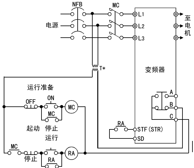
变频器的启停回路例
