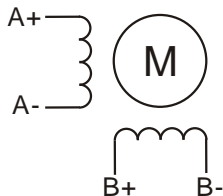
两相电机四引线
