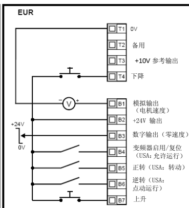
图 6-6 Pr05 = E.Pot
