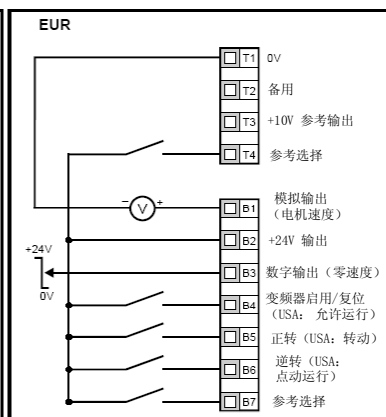
图 6-4 Pr05 = Pr
